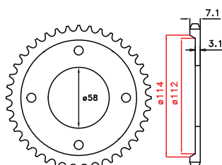
รุ่น : WAVE(428) จำนวนฟัน : 34T เบอร์โซ่ : 428 เจาะรูสกรู : Ø8.5x4x90
