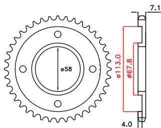
รุ่น : WAVE(428) จำนวนฟัน : 36T เบอร์โซ่ : 428 เจาะรูสกรู : Ø8.5x4x90
